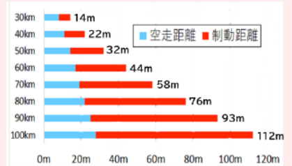
・速度による停止距離の変化
